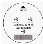
Modelo de furação (x1)
